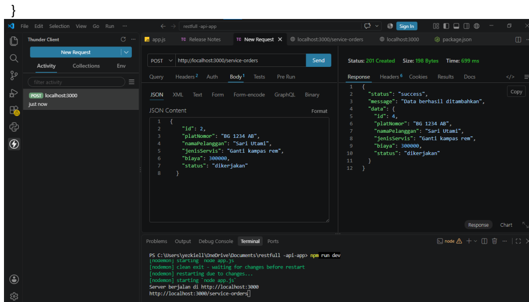
Gambar 6. Pengujian POST data pelanggan.
