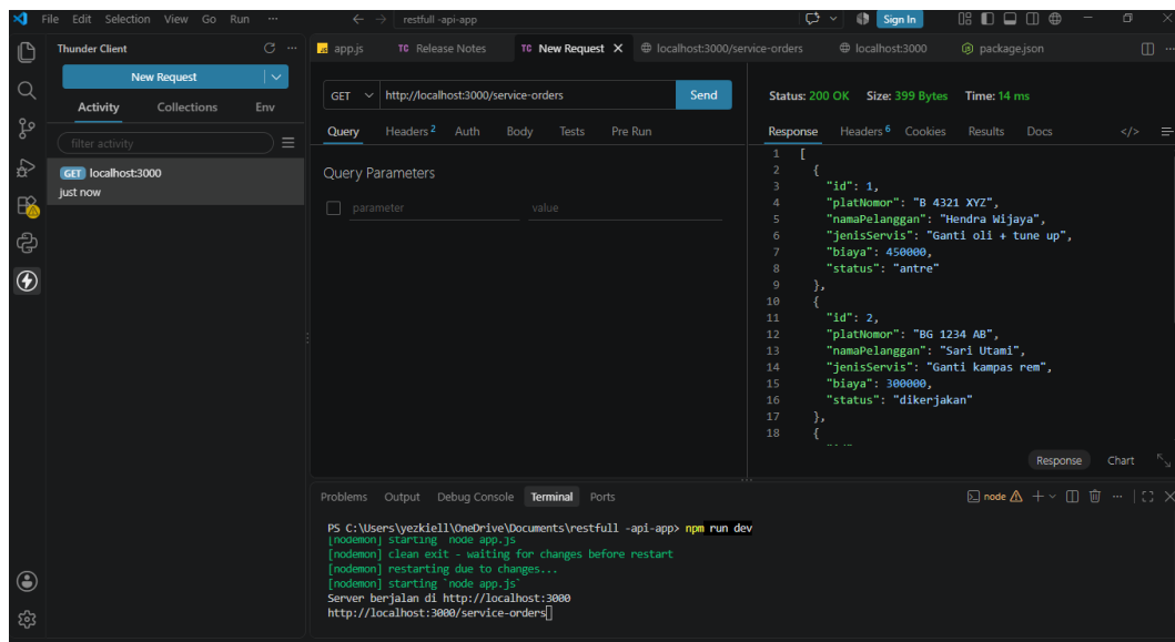
Gambar 2. Pengujian GET //service-orders/ menggunakan Thunder Client.
