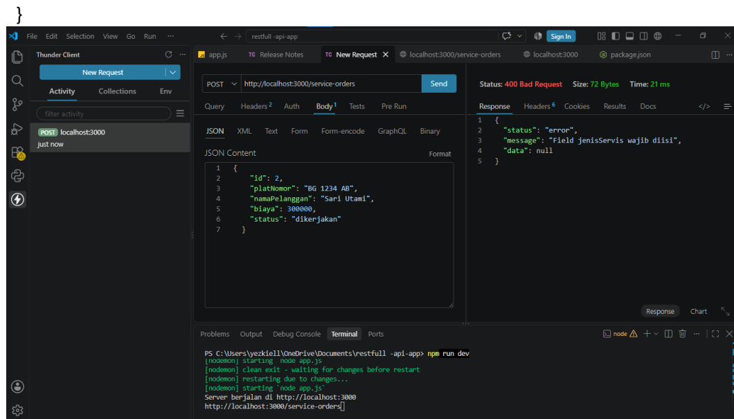
Gambar 7. Pengujian POST dengan data tidak lengkap.
